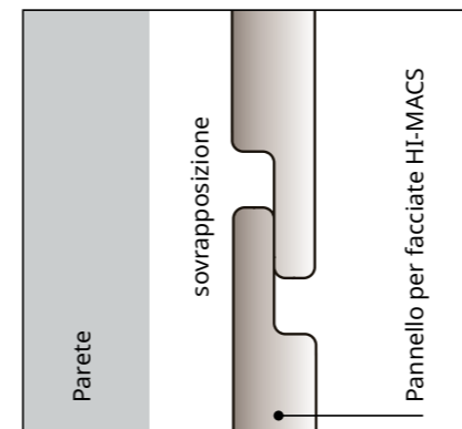
Pannelli sovrapposti
